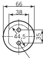
Отверстия для крепления на панель
