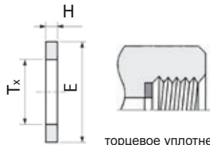
торцевое уплотнение для штуцеров типа CGC
