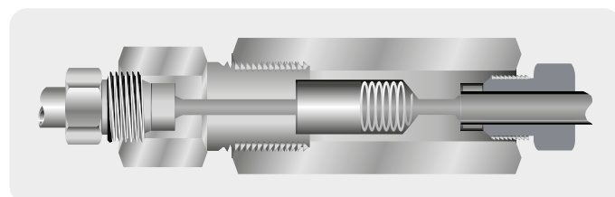
Фильтр с фильтрующим элементом типа "чаша"
